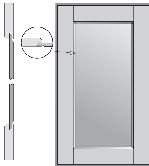
Door Cross Section
